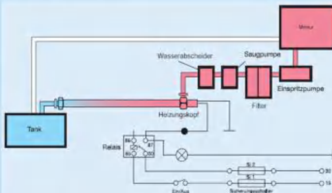
Typisches Einbauschema
